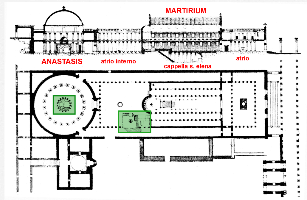
PIANTA E SEZIONE DEL SANTO SEPOLCRO DI GERUSALEMME (fine IV secolo)
